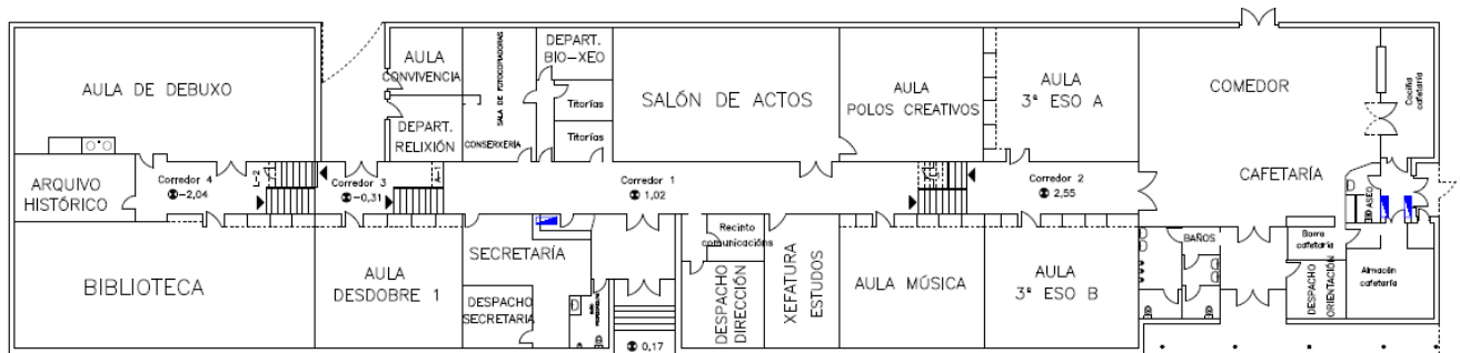
Planta baixa - Edificio principal
