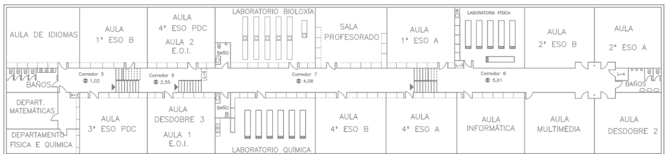
Planta primeira - Edificio principal
