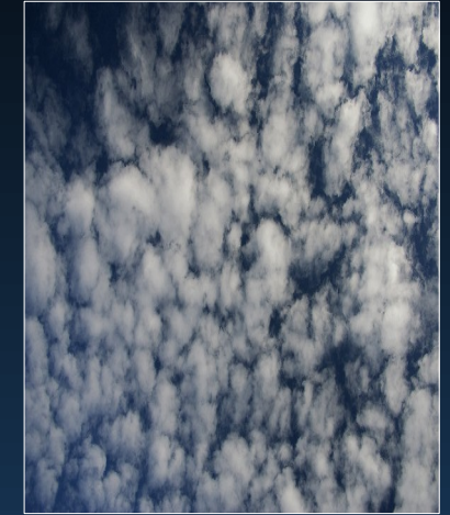
Cirrostratus
