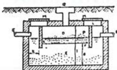
FIG. 1. Fosa séptica de un compartimento
