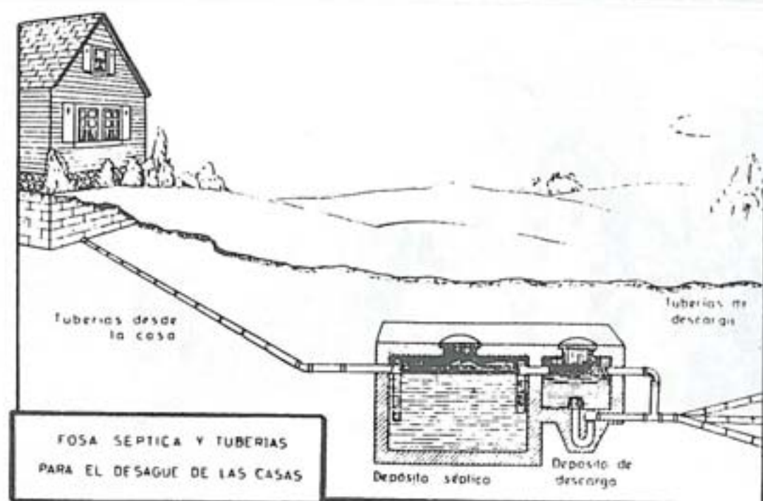
Fig. 3. Evacuación de excretas en zonas rurales. (Monografía de la O.M.S.)
