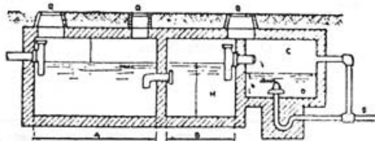
FIG. 2. Fosa séptica de dous compartimentos
