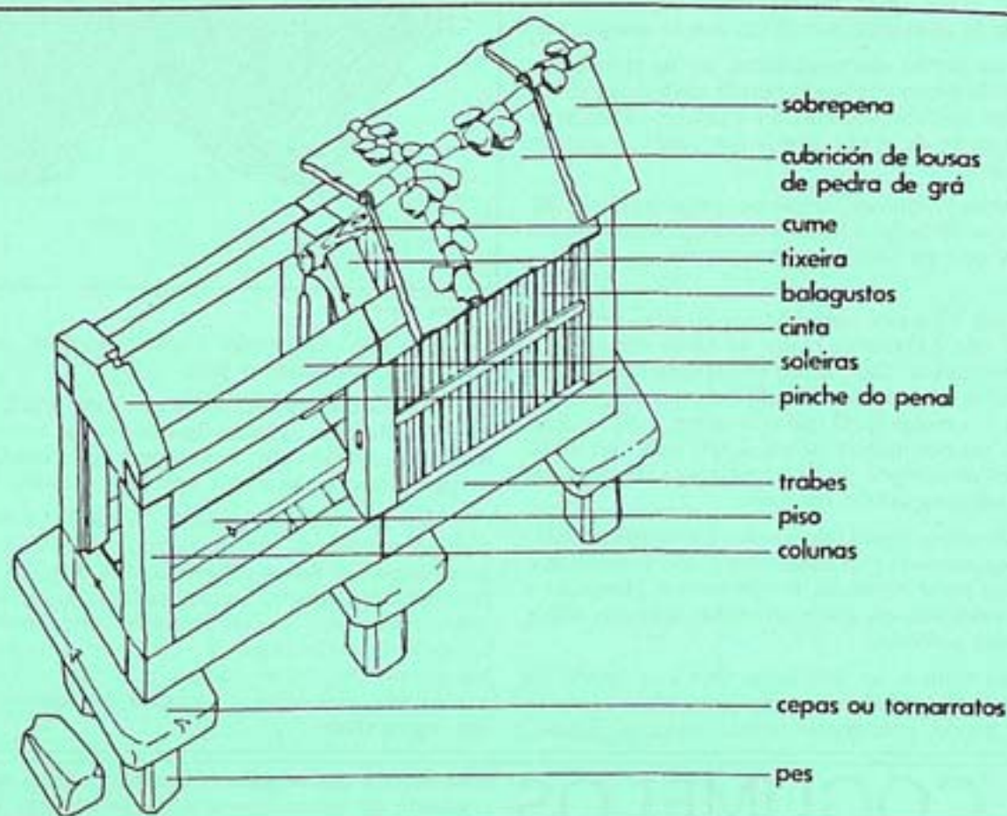
Esquema descriptivo dos principais elementos do hórreo.
