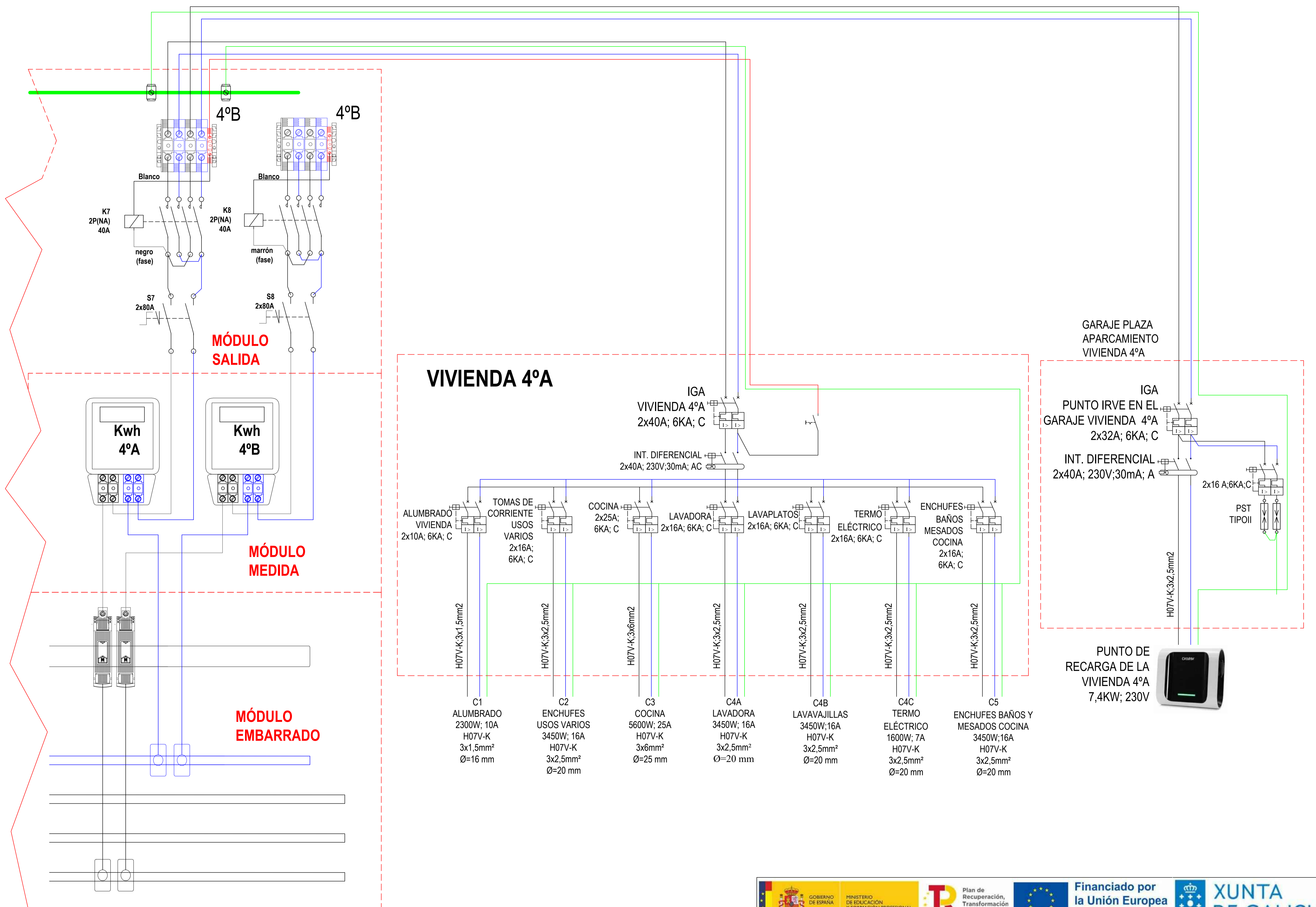
ESQUEMA DE CENTRALIZACIÓN PARA 8 SUMINISTROS MONOFÁSICOS CON IRVE INDIVIDUAL VÁLIDO PARA ESQUEMAS 2 3A 3B y 4A DE LA ITC-BT-52 DEL REBT
