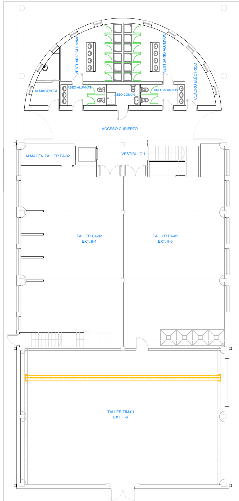
PLANTA BAJA EDIFICIO ANEXO II
