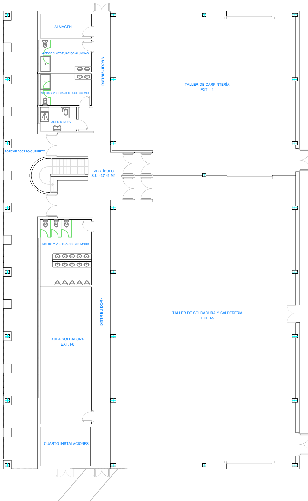
PLANTA BAJA EDIFICIO ANEXO I
