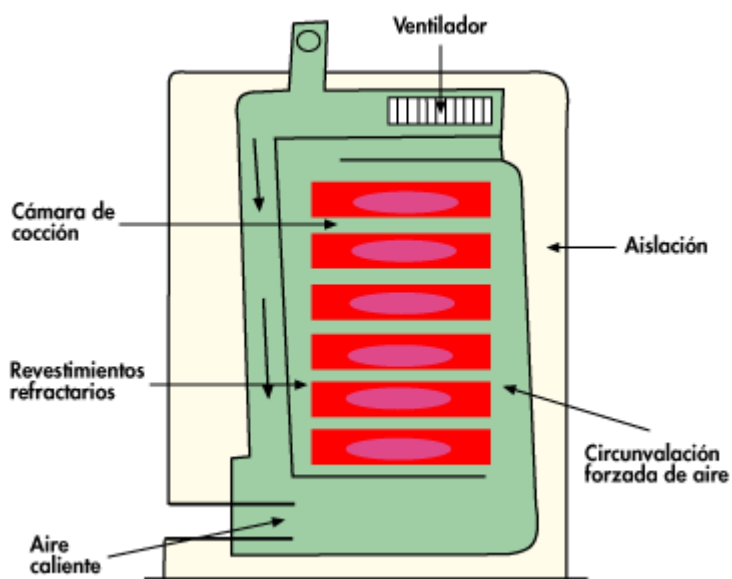
GRÁFICO 2 / ESQUEMA DE UN HORNO DE TUBOS ANULARES
