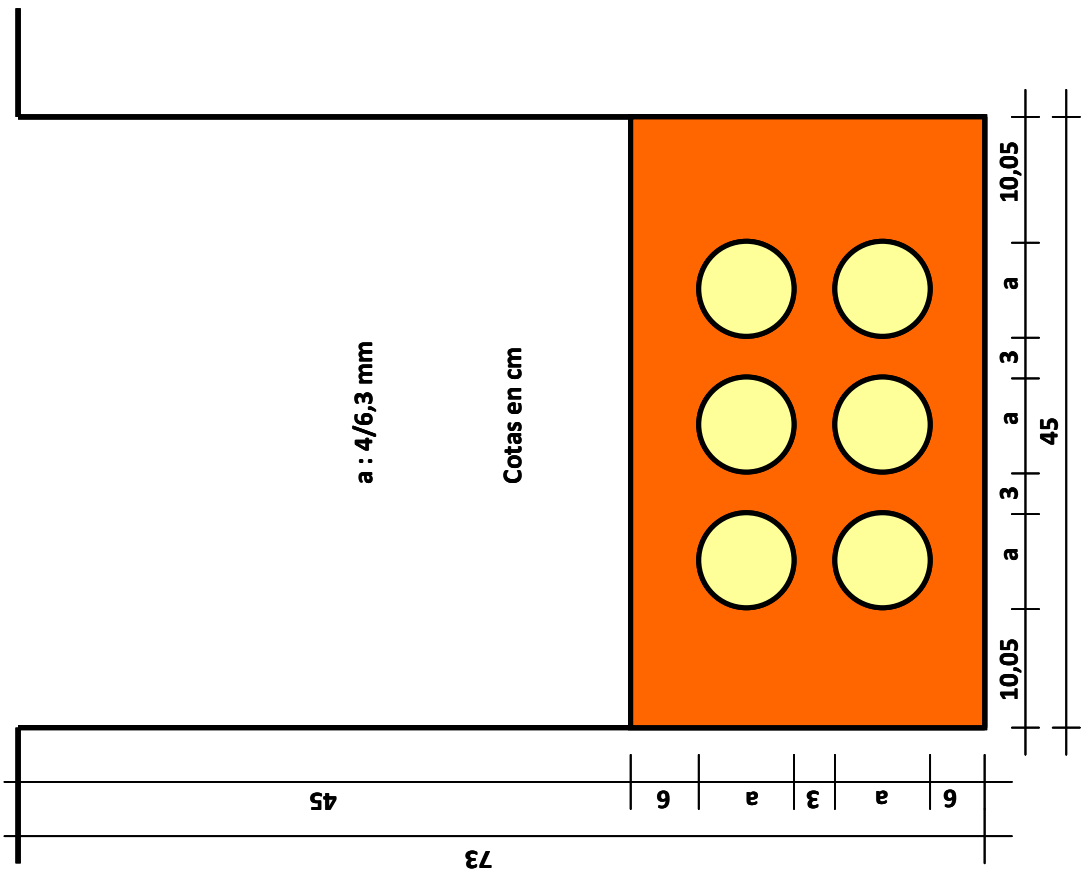
APENDICE 4: Sección transversal de la canalización de enlace
