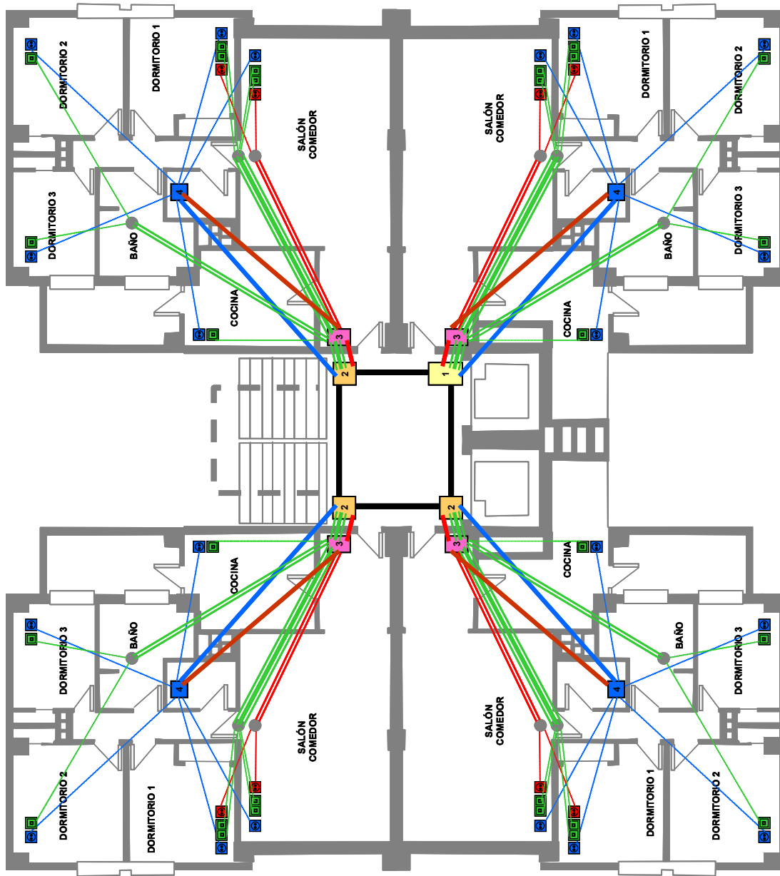
APENDICE 7: Canalización secundaria y red interior de usuario
