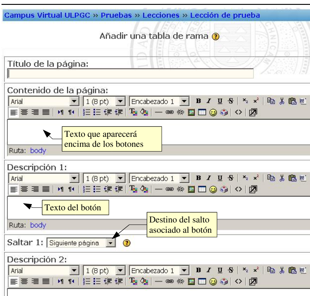
Figura 58. Edición de una tabla de ramificación de una lección
