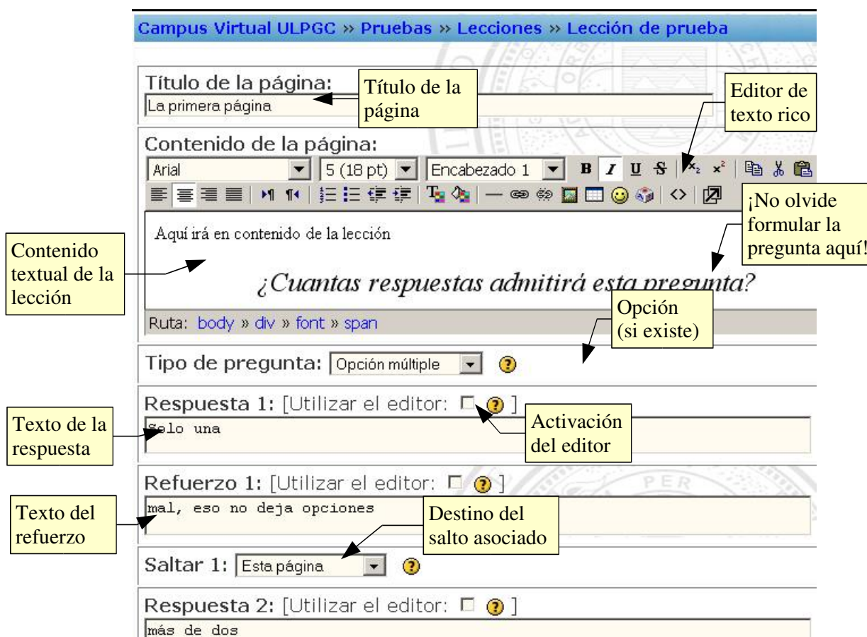
Figura 56. Edición de una página de preguntas de una lección
