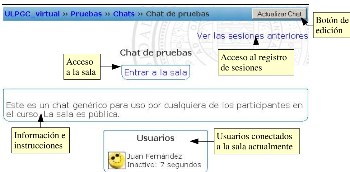
Figura 26. Página de acceso a la sala de chat
