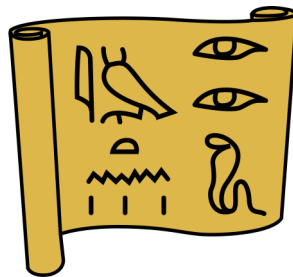
jerooglífico
