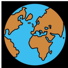
La Tierra
