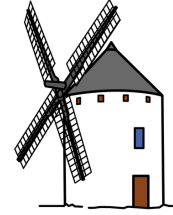
molino
