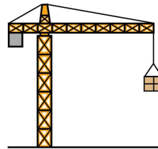
grúa
