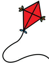
cometa
