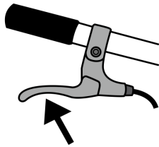
freno
