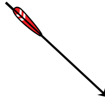
flecha
