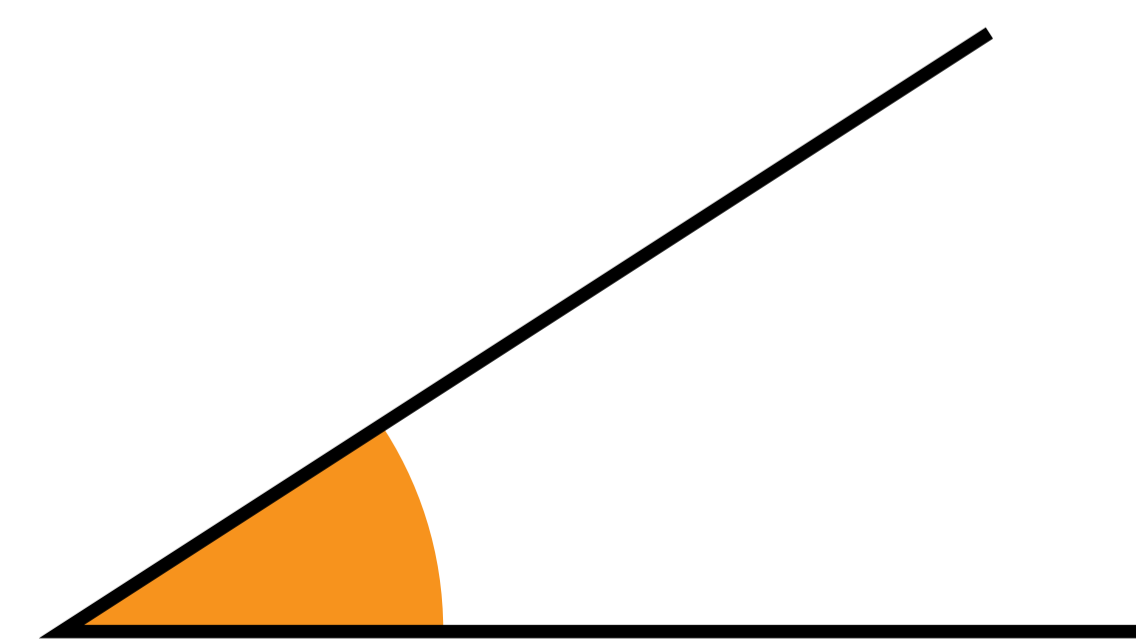
ÁNGULO AGUDO
