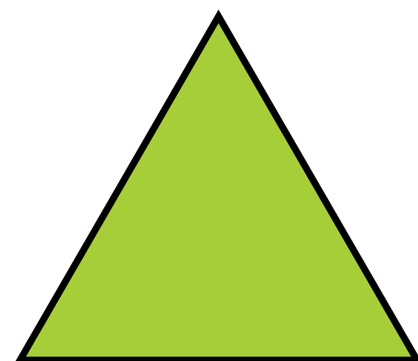
TRIÁNGULO
