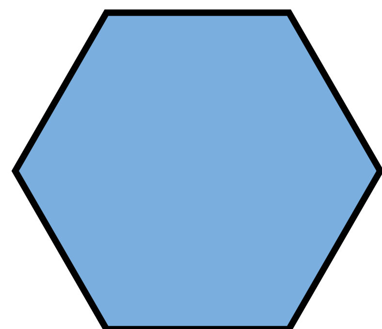
HEXÁGONO
