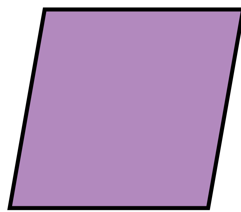
CUADRILÁTERO
