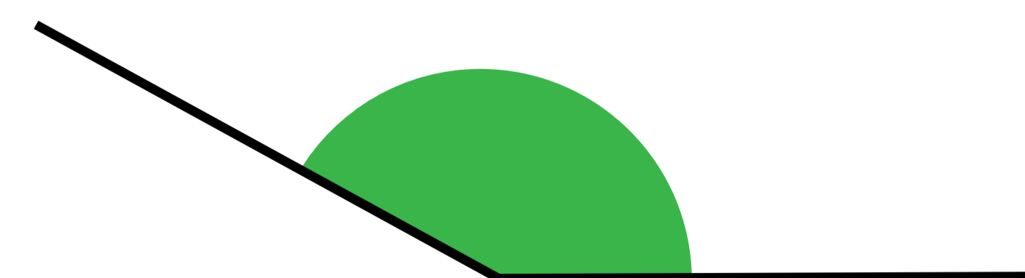
ÁNGULO OBTUSO
