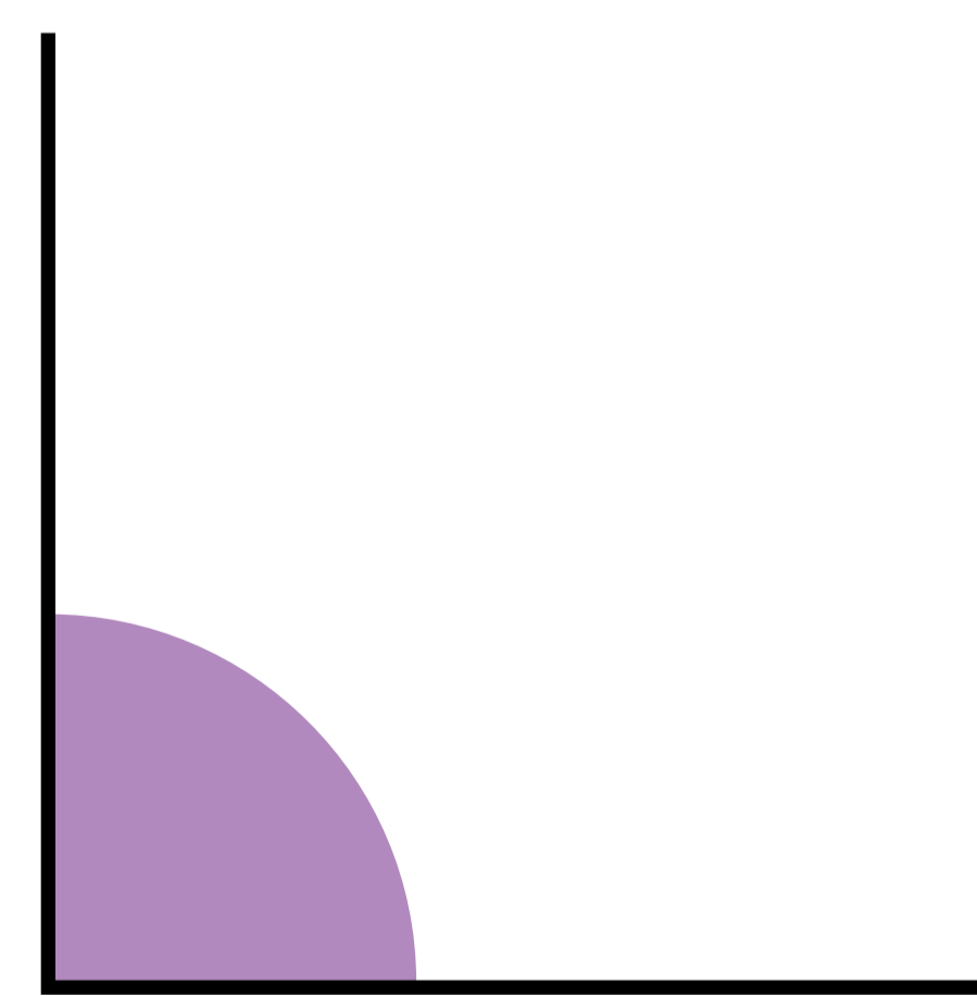
ÁNGULO RECTO
