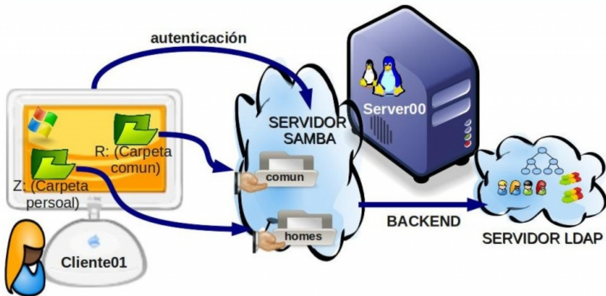
Escenario 4.1: Configuración de servidor samba e clientes Windows
